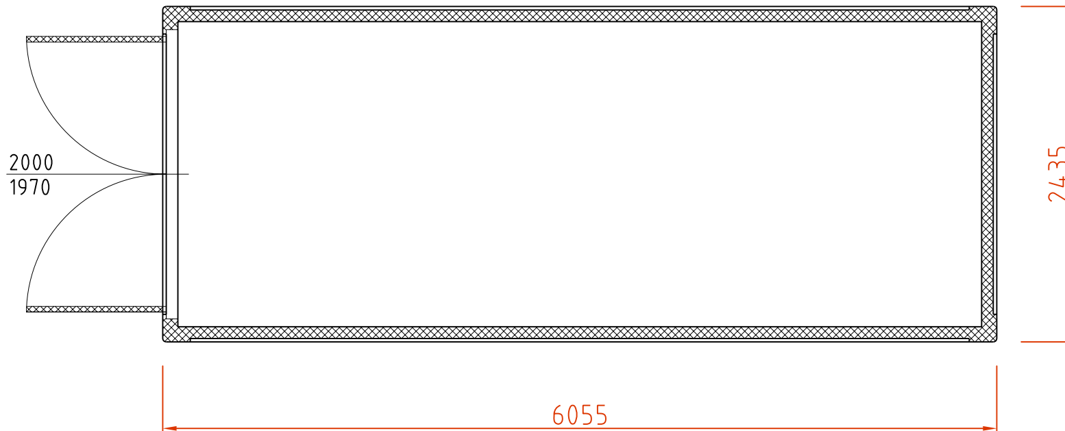
DVOUKRIDLE OCELOVE DVERE 2000x1970mm ZATEPLENE
