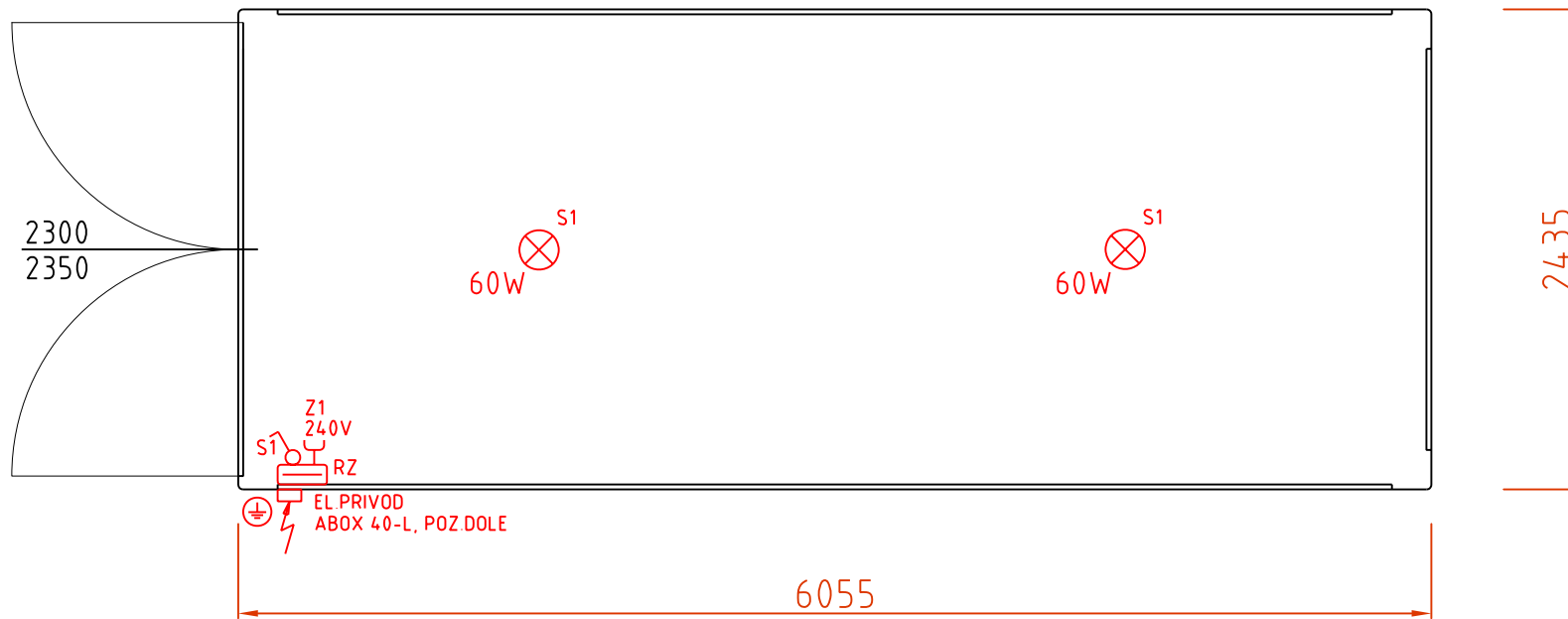
DVOUKRIDLA OCELOVA VRATA 2300x2350mm S TYCOVYM ZAVIRANIM
