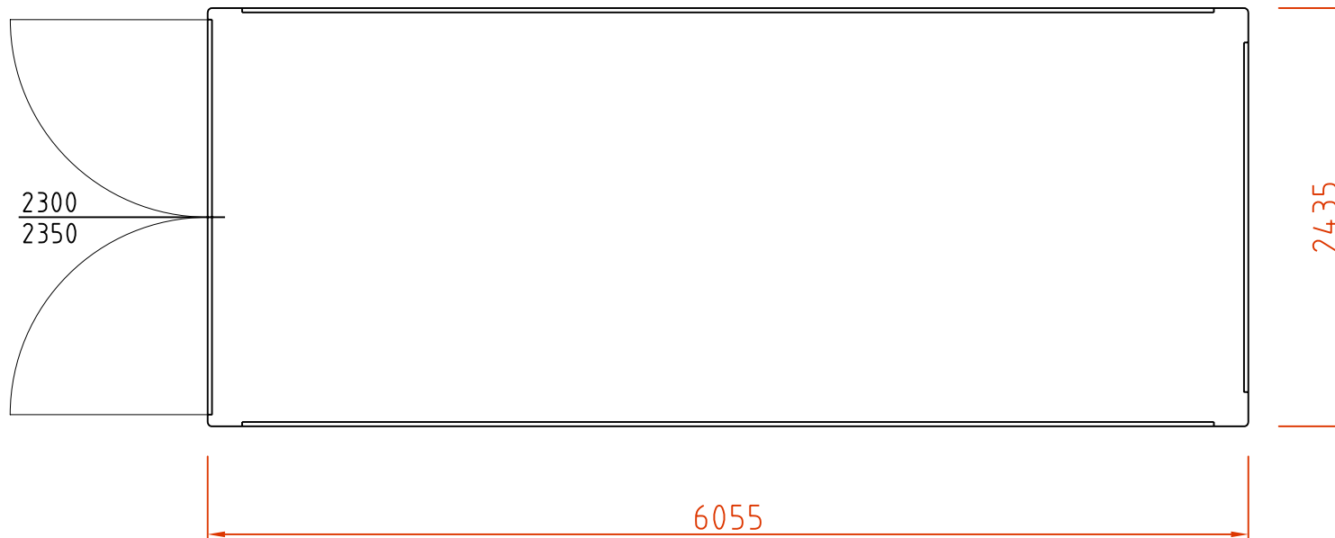
DVOUKRIDLA OCELOVA VRATA 2300x2350mm S TYCOVYM ZAVIRANIM
