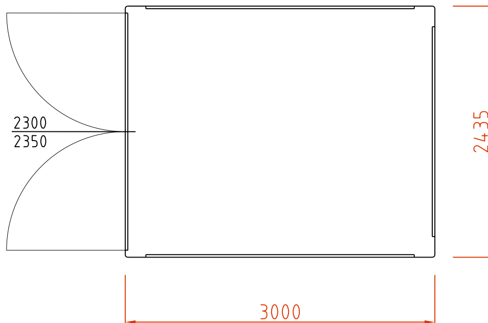
DVOUKRIDLA OCELOVA VRATA 2300x2350mm S TYCOVYM ZAVIRANIM
